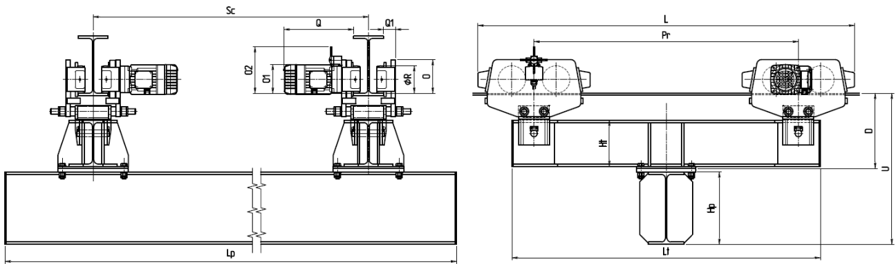
Pont suspendu DPS3 – Capacité de charge 3200 kg – Palan DMK
