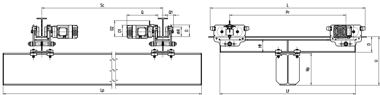
Pont suspendu DPS1 – Capacité de charge 1000 kg – Palan DRH1
