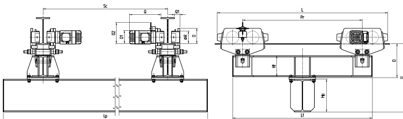
Pont suspendu DPS3 – Capacité de charge 3200 kg – Palan DRH1
